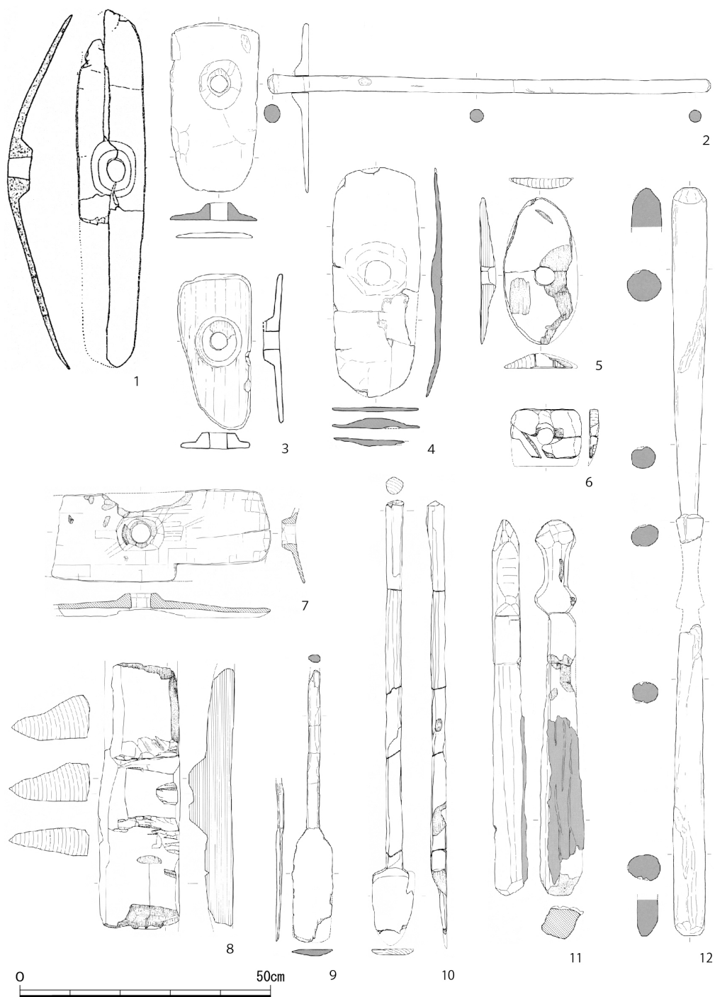
図27 北部九州における刻目凸帯文土器(夜臼式)~弥生時代前期前葉(板付Ⅰ式)の木製農具 (1:福岡市 鶴町, 2・4・9・12:福岡市 雀居4次調査, 3・7:唐津市 菜畑, 5・6・8・10:福岡市 橋本一丁田2次調査, 11:福岡市 雀居5次調査)
