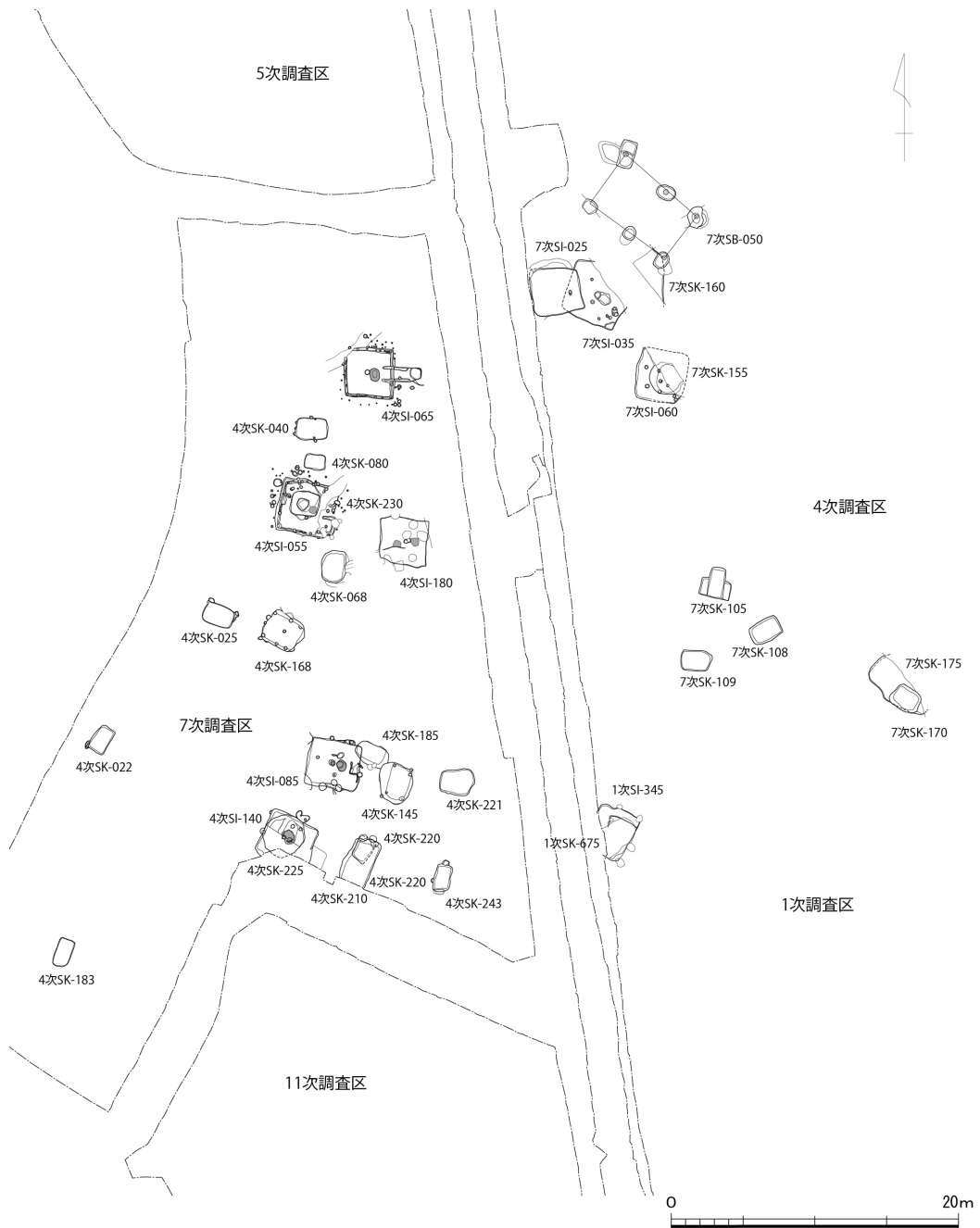
図10 福岡県太宰府市前田遺跡の弥生時代前期初頭～中葉(板付Ⅰ～Ⅱ式古段階)の集落(縮尺1/400)
