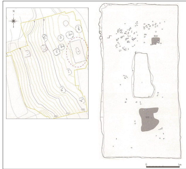
圖 7. 김제 수록리 1호 주거 (군산대학교박물관 2014:74 필자 재편집)
