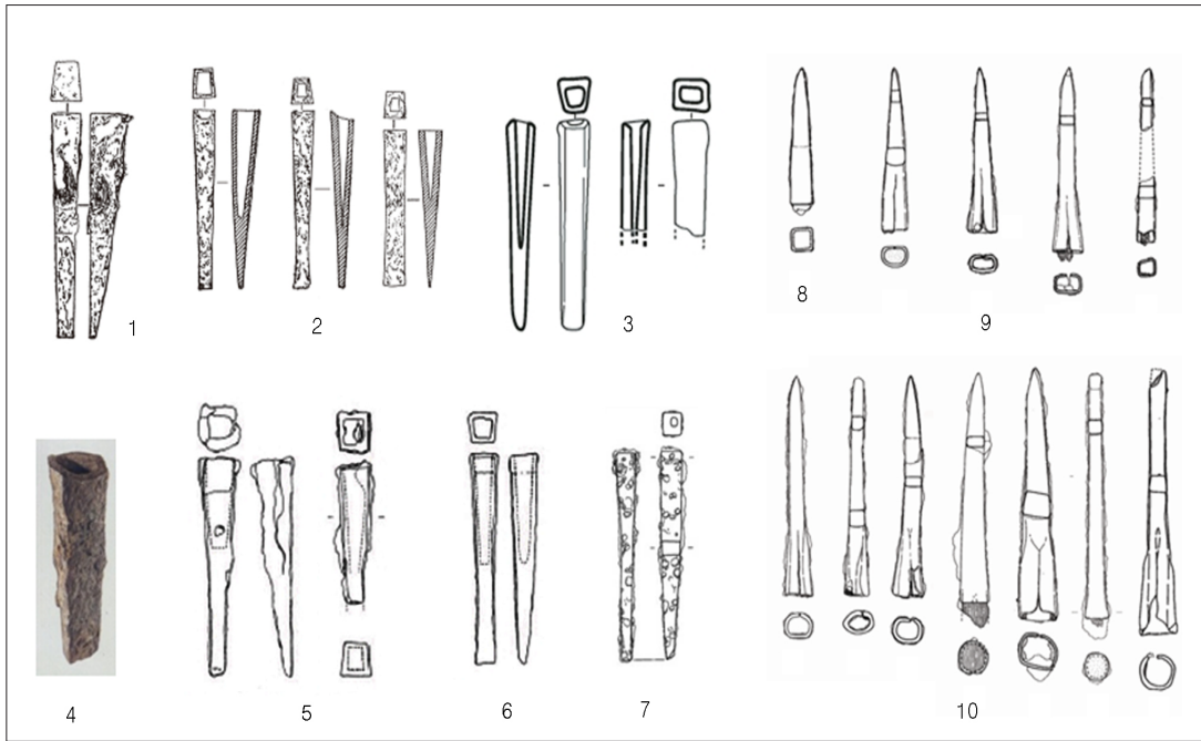
〈그림 10〉 하북·요령·서북한·남부지방 출토 철착(촉척 부동)
